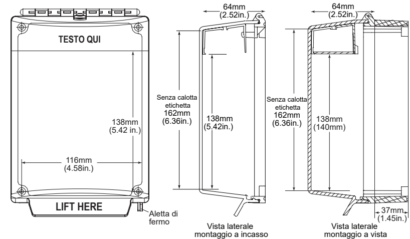
Dimensioni prodotto
